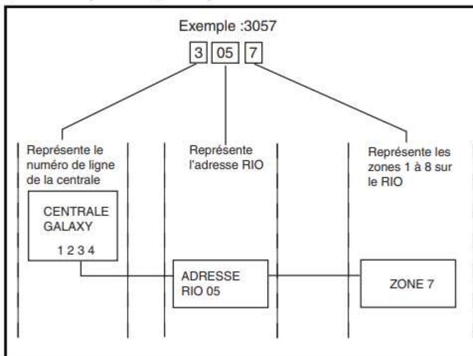
Figure 2-9. Adresses de zones
