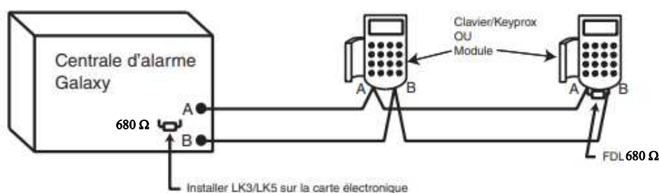
Figure 2-6. Configuration en guirlande
