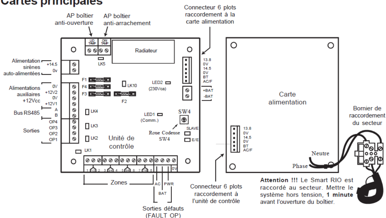
Figure 3. Carte Smart RIO EN F.
