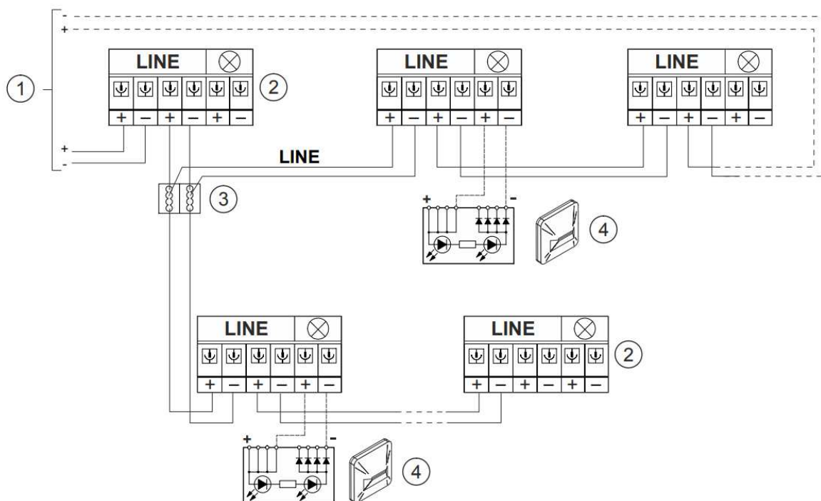
Figure 12: Schéma de raccordement pour ligne de détection adressée avec et sans indicateurs d'action externes (sans câbles blindés)
