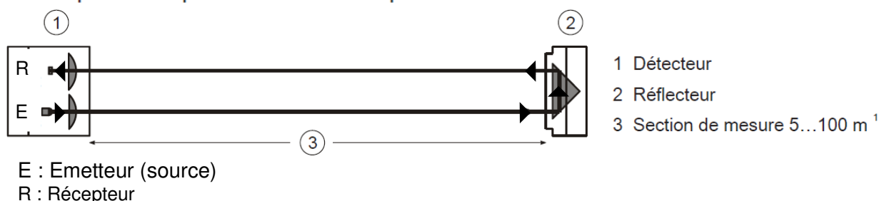
Figure 1: Fonctionnement du détecteur linéaire de fumée sans fumée
