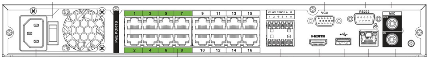
Façade arrière de l'enregistreur
