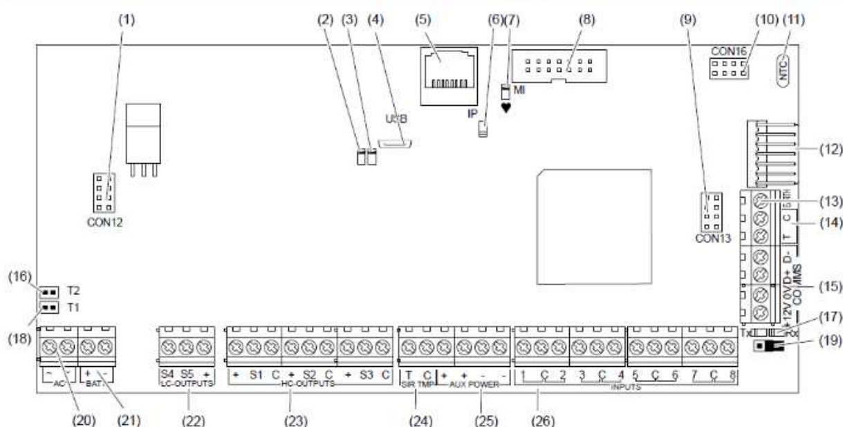
Figure 9 : Présentation d'Advisor Advanced ATsx500A(-IP)
