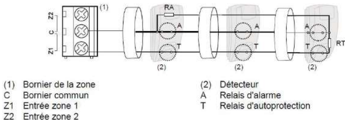
Figure 18 : Boucle double
