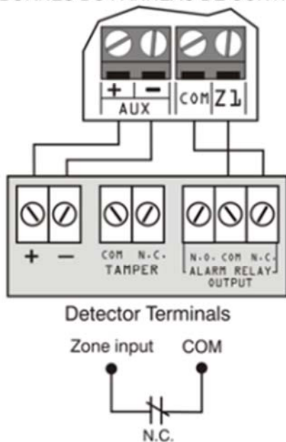
Contact N.F. sans résistance d'EDL BORNES DU PANNEAU DE CONTRÔLE
