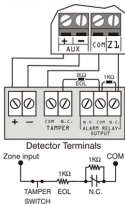
N.C, avec EDL, avec autoprotection & reconnaissance de sabotage BORNE DU PANNEAU DE CONTRÔLE
