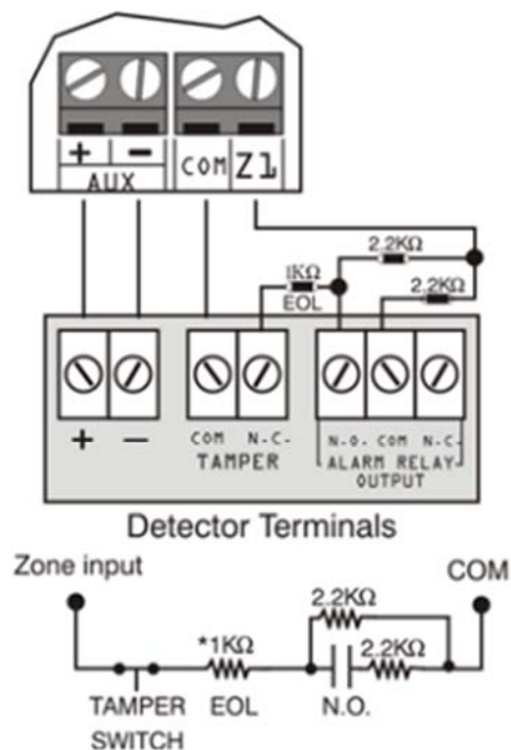
N.O, avec EOL, avec autoprotection & reconnaissance de sabotage BORNE DU PANNEAU DE CONTRÔLE
