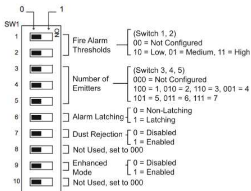
Figure 4-7: Interrupteur DIP
