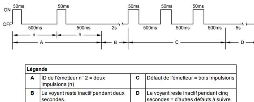
Figure 2-3: Défaut d'émetteur
