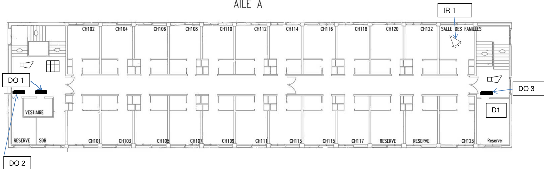
Plan du site intrusion étage « GROUPE 3 »
