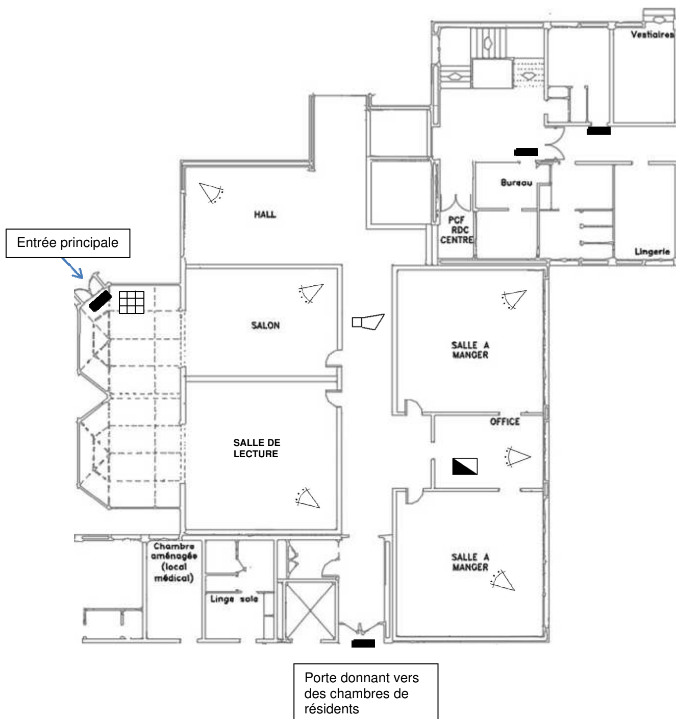
Plan du site intrusion rez-de-chaussée « GROUPE 2 »
