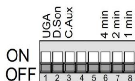
Dipswitch de paramétrage de l'UGA
