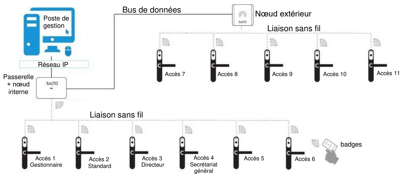
Synoptique de l'installation
