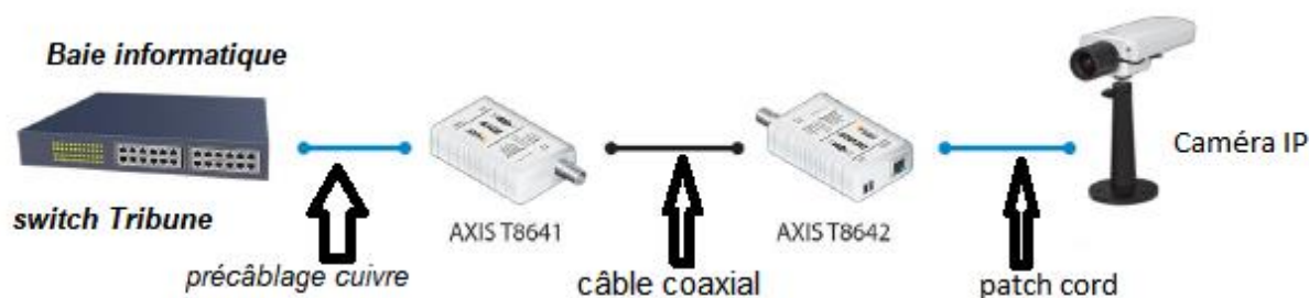
Schéma de la liaison
