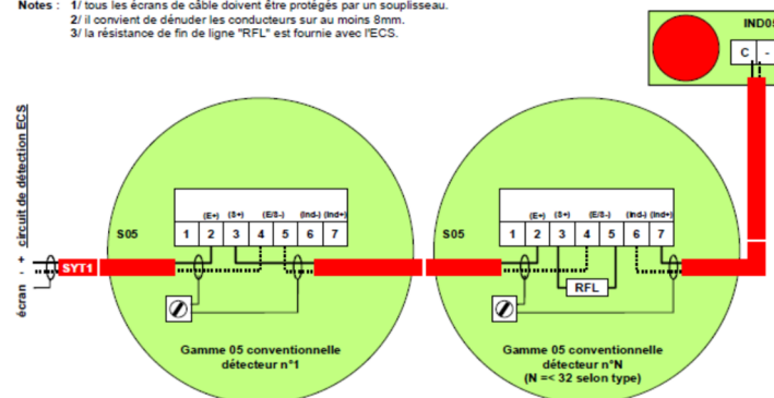
CIRCUIT OUVERT DE DETECTION : DETECTEURS AUTOMATIQUES
