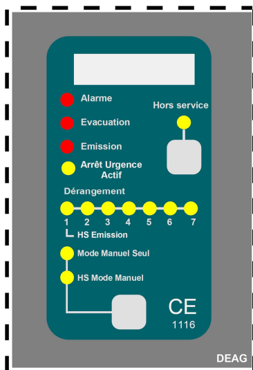
Face avant centrale ALPHA E2/2/10
