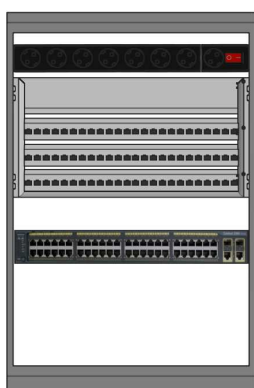
Baie du sous-répartiteur SR7 COMM7-1 ref : WS-C2960-48PST-L
