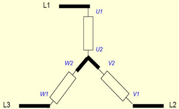
Couplage Etoile
