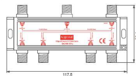
Répartiteur 6 directions = 117,5 x 60,1 x 17,4
