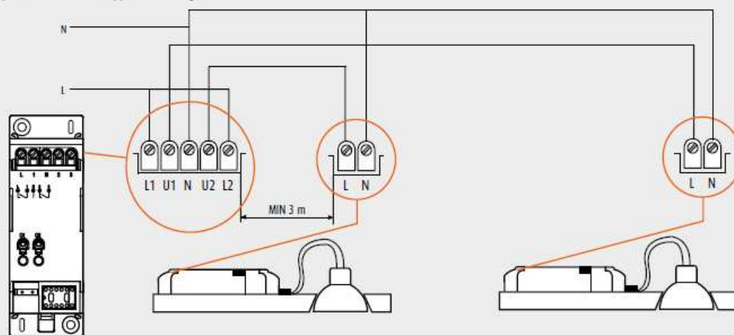
Schéma pour le raccordement d'appareils d'éclairage
